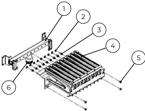
Рис. 39. Газовая горелка.
