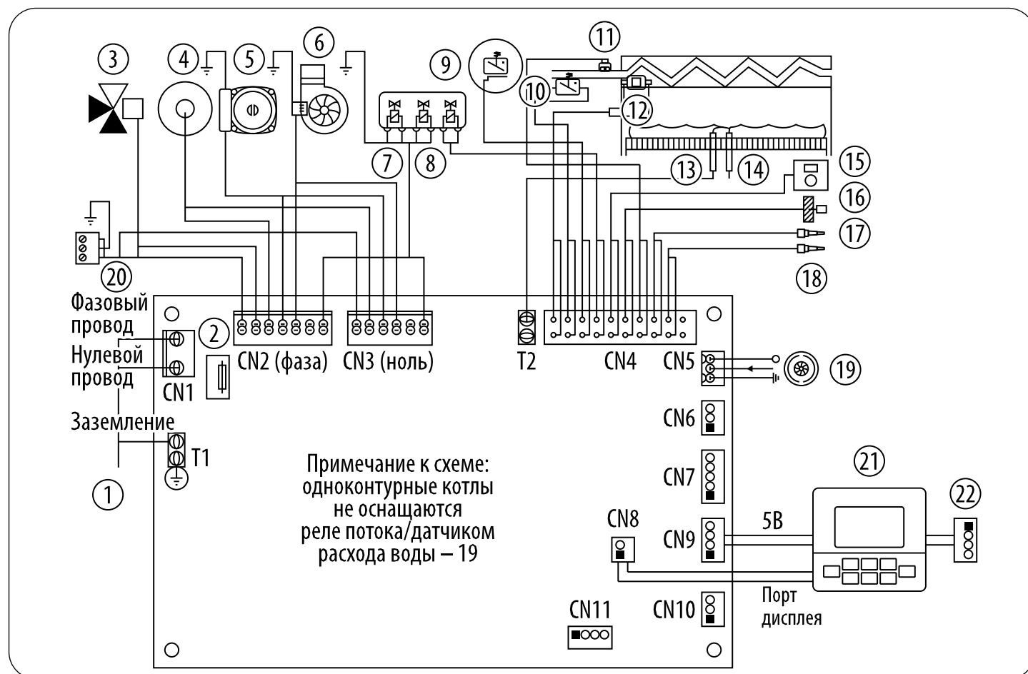
Рис. 46. Электрическая схема.
