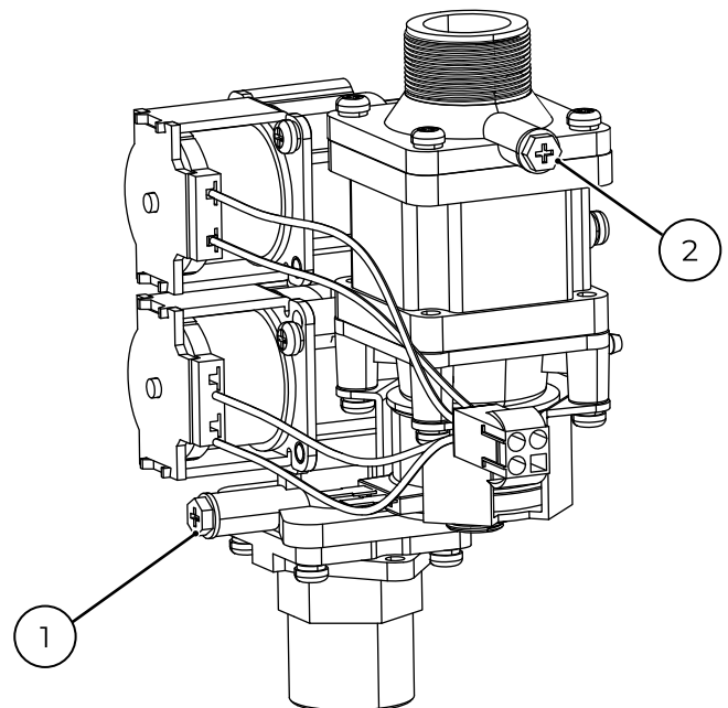
Рис. 40. Газовый клапан.
