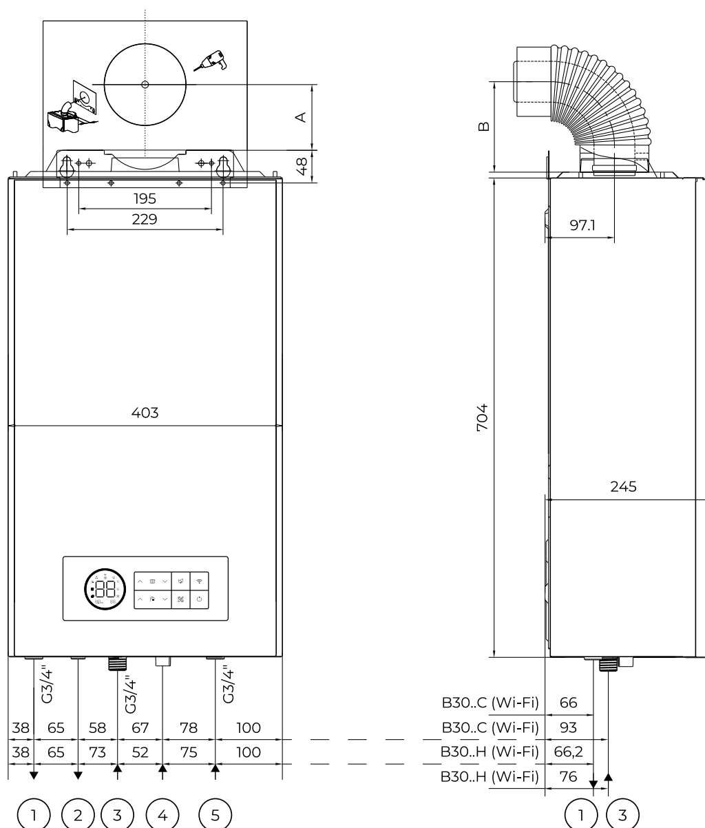
Рис. 42. Монтажные размеры B30 18 C/H (Wi-Fi), B30 24 C/H (Wi-Fi).
